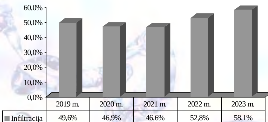
8 pav. Infiltracija į nuotekų tinklus
