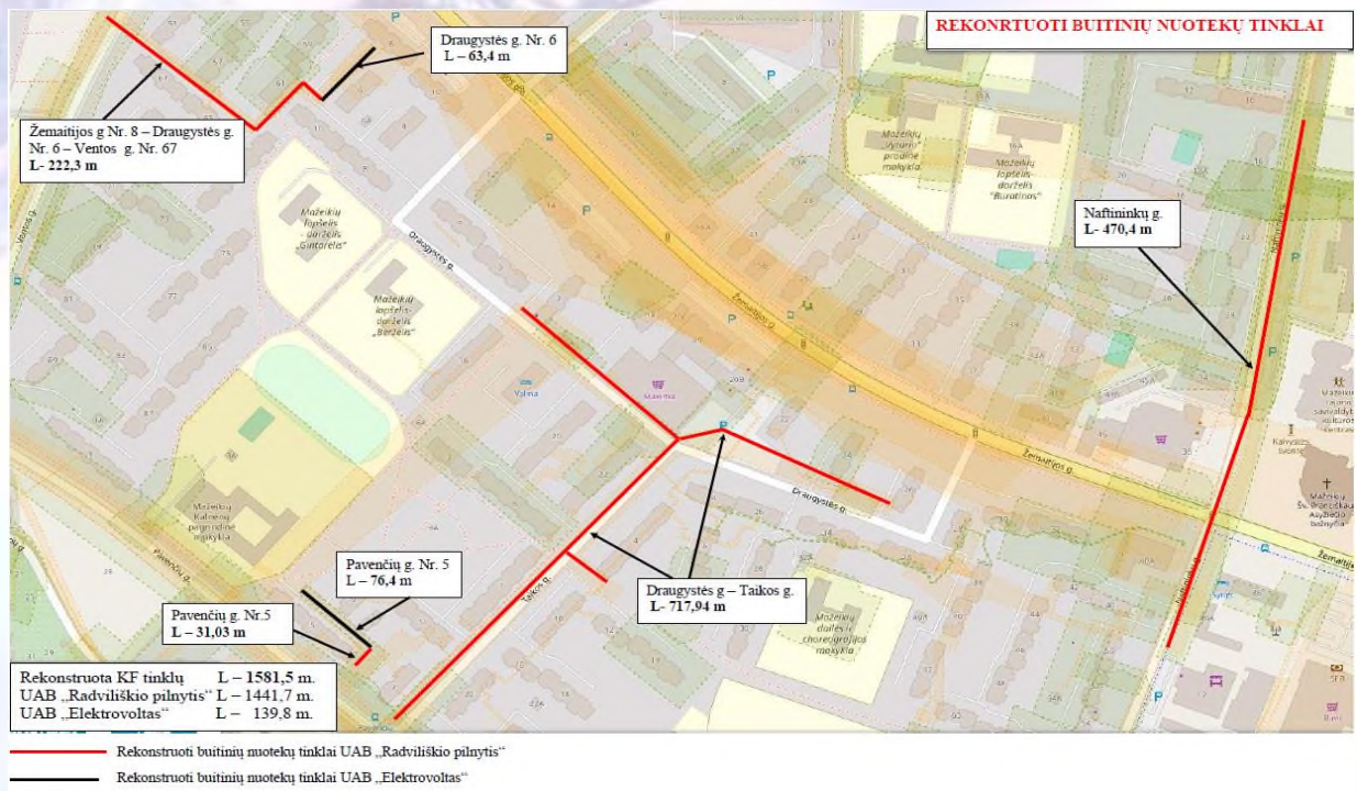
35 pav. Buitinių nuotekų tinklų rekonstravimas Žemaitijos, Ventos, Naftininkų, Pavenčių, Taikos, Draugystės g., Mažeikių m.
