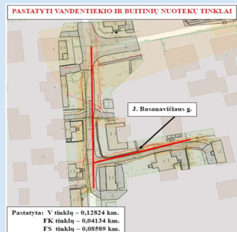
V, N tinklų vietos schema
