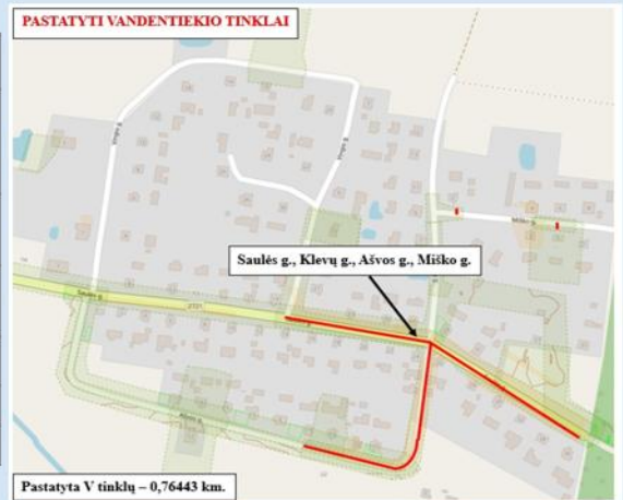
V tinklų vietų schema
